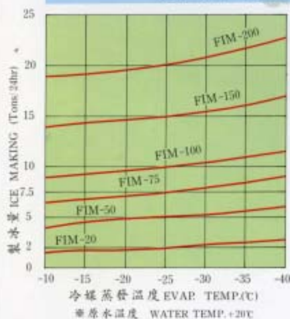
製冰能力曲線圖
